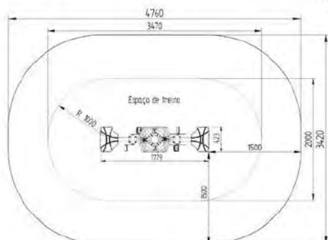
BIO0001 Bicicleta Doble 01
