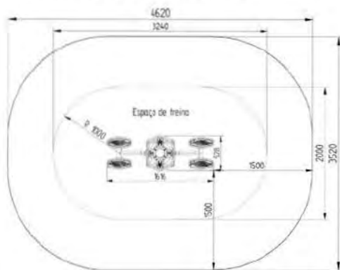
BIO0005 Surf Doble 05
