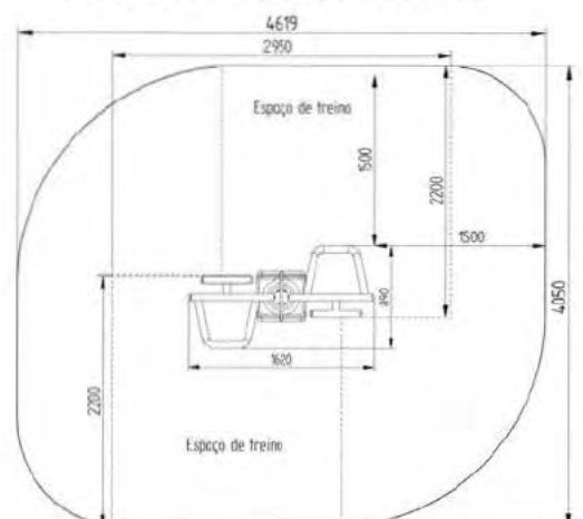
BIO0006 Abdominal Doble 06
