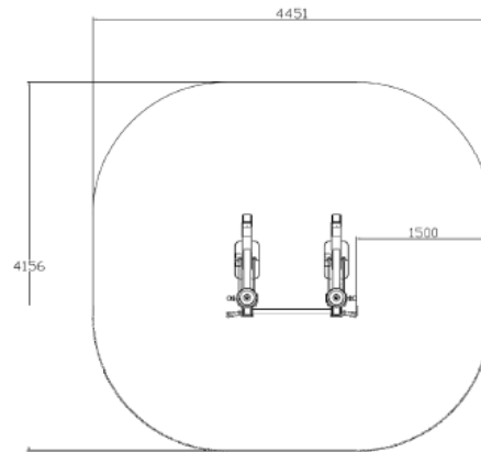
PRO0001 Extensión de Cuádriceps
