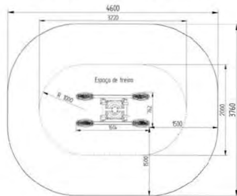
BIO0004 Esquí Doble 04
