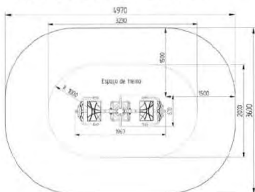
BIO0008 Columpio Doble 08
