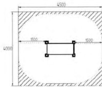
STW0001 Banco de Abdominales 01
