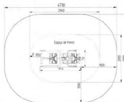
BIO0007 Ascensor + Piernas 07
