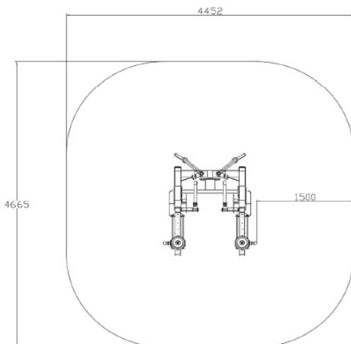
PRO0002 Contractora Pectoral
